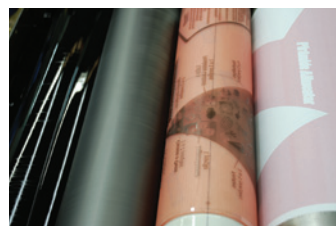
Figura 6 - Impressora flexográfica – sistema convencional (doctor-roll): detalhe de um cilindro entintador, anilox e cilindro porta-clichê de fotopolímero de uma máquina flexográfica no momento da impressão.
