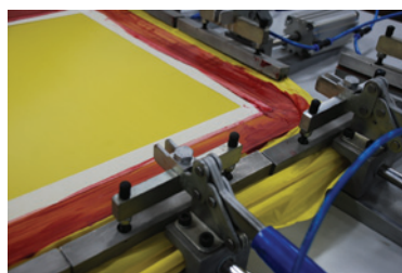
Figura 8 - Forma serigráfica – Etapa de confecção de uma tela serigráfica, quando o tecido é tensionado por meio de pinças pneumáticas e fixado ao quadro, utilizando-se um adesivo.
