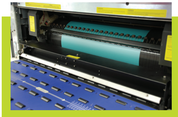
Figura 2 - Gravadora de chapas offset – Chapa para impressão offset no interior de uma máquina do sistema computer-to-plate, antes do processamento
