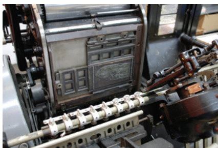
Figura 7 - Impressora tipográfica – Detalhe de uma máquina de impressão tipográfica, exibindo a fôrma de impressão, o clichê, fixo à rama através de guarnições.
